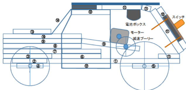
組立図
