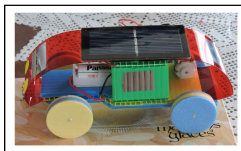
写真2) 試作機3号
